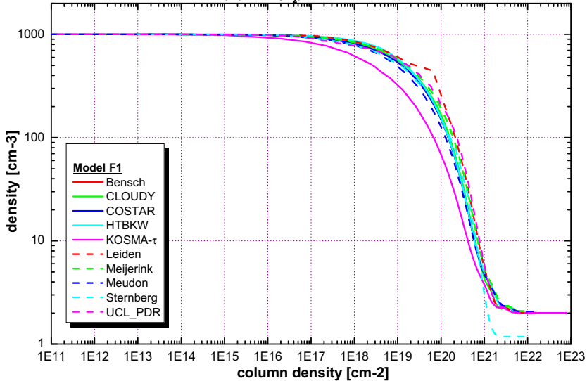
n(\text{H}) vs N(\text{H}_2) - n=10^3 \text{ cm}^{-3} , \chi=10
