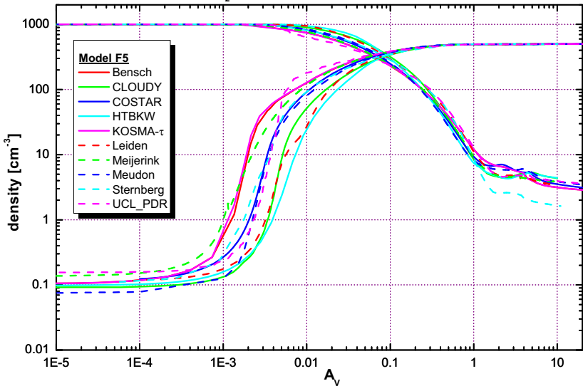
H and H 2 density - n=10^3 \text{ cm}^{-3} , \chi=10^1 , variable T
