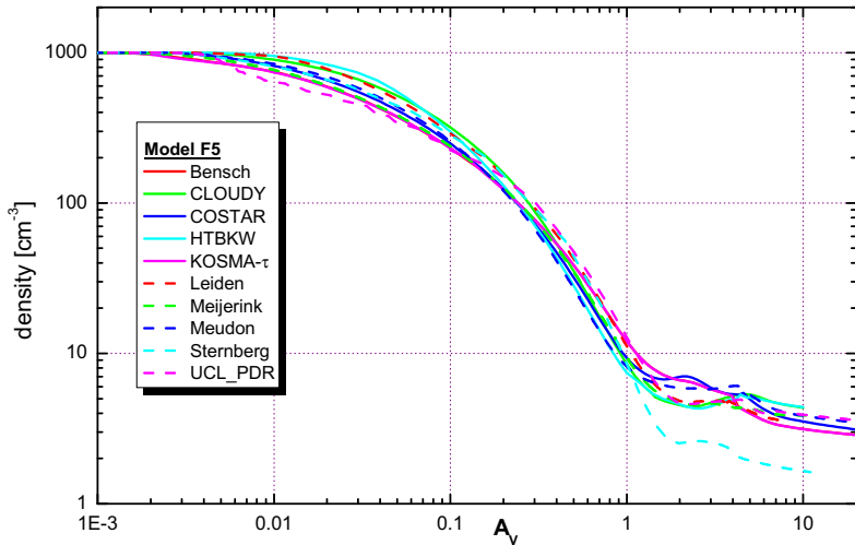
H density - n=10^3 \text{ cm}^{-3} , \chi=10^1 , variable T
