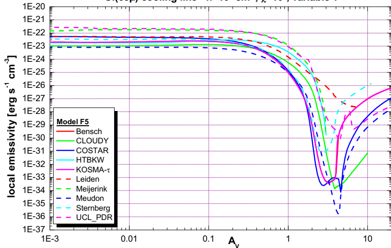
OI(63 \mu ) cooling line - n=10^3 \text{ cm}^{-3} , \chi=10^1 , variable T
