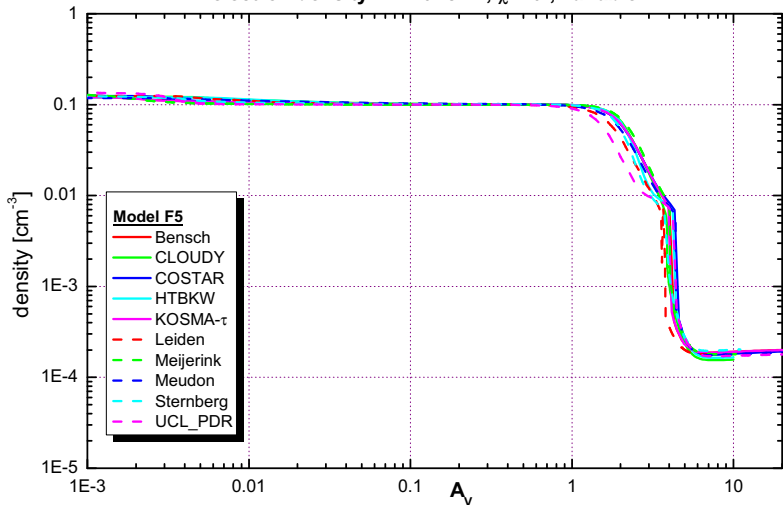
electron density - n=10^3 \text{ cm}^{-3} , \chi=10^1 , variable T
