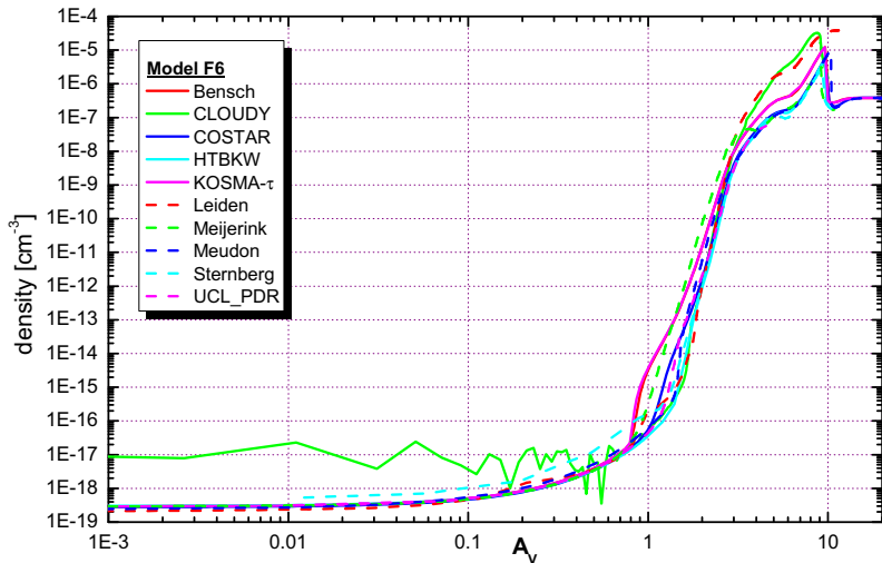
CH density - n=10^3 \text{ cm}^{-3} , \chi=10^5 , variable T
