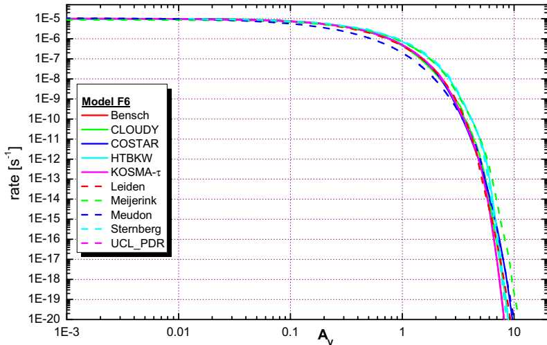
CO dissociation rate - n=10^3 \text{ cm}^{-3} , \chi=10^5 , variable T
