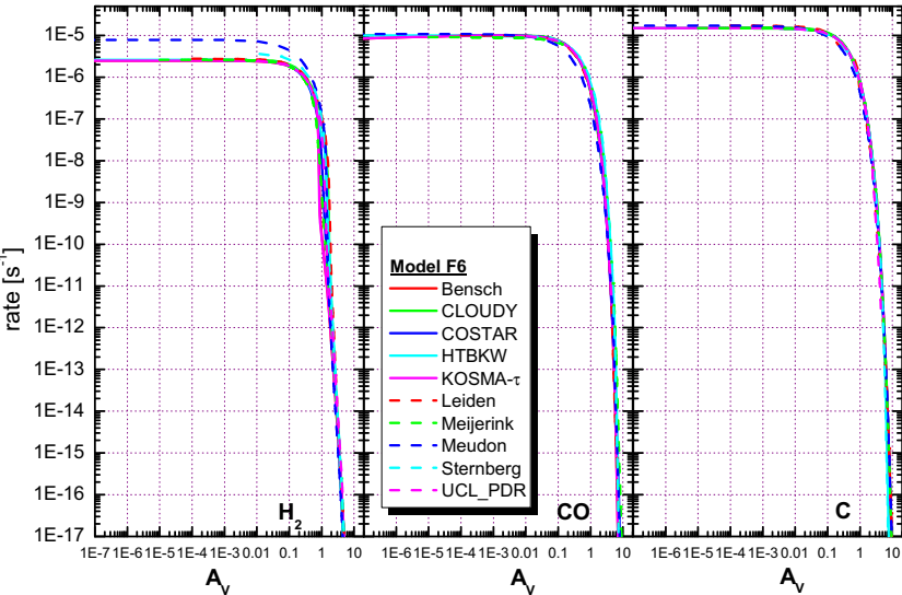
photo rates - n=10^3 \text{ cm}^{-3} , \chi=10^5 , variable T
