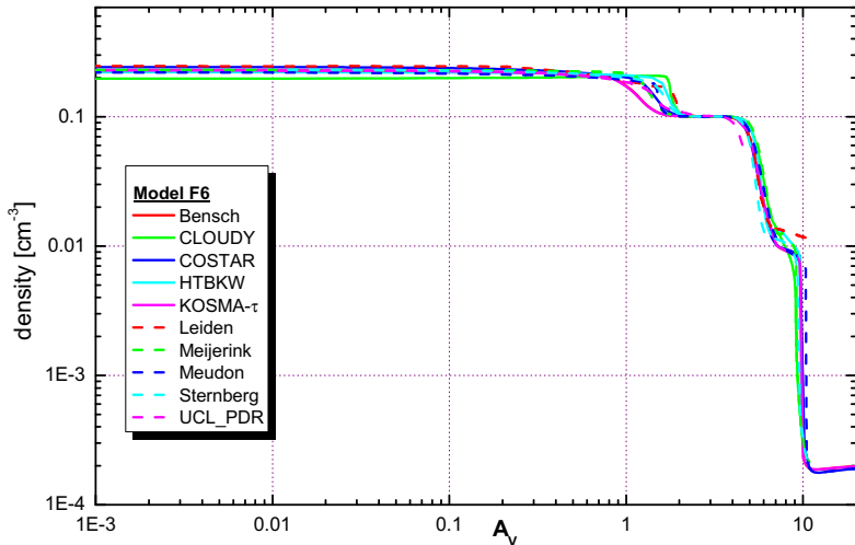
electron density - n=10^3 \text{ cm}^{-3} , \chi=10^5 , variable T
