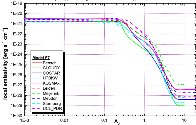
Cl(370 \mu ) cooling line - n=10^{5.5} cm ^{-3} , \chi=10^1 , variable T
