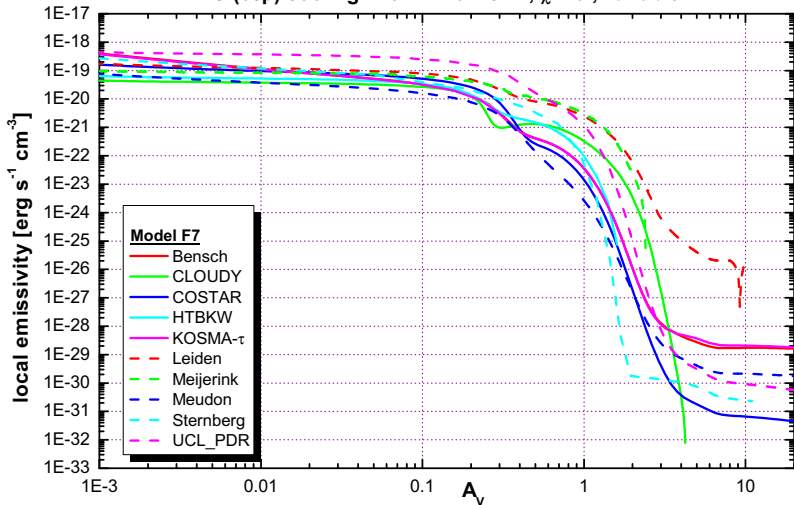
OI(63 \mu ) cooling line - n=10^{5.5} cm ^{-3} , \chi=10^1 , variable T
