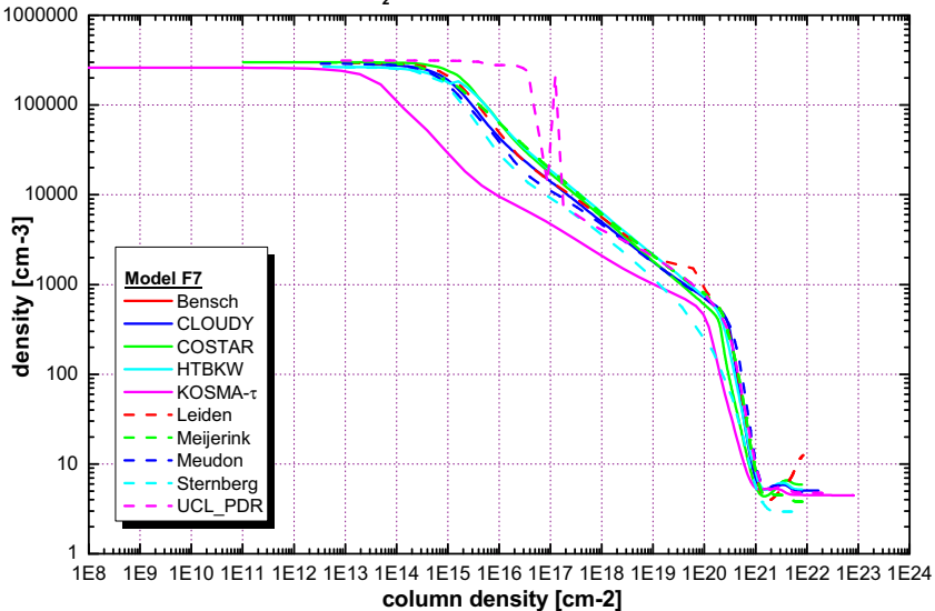
n(H) vs. N(H_2) - n=10^{5.5} \text{ cm}^{-3} , \chi=10^1 , variable T
