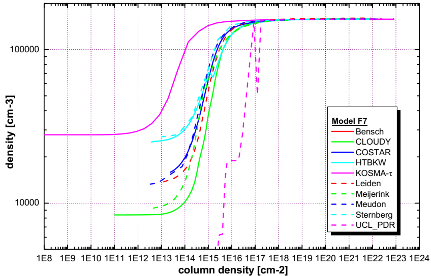
n(\text{H}_2) vs. N(\text{H}_2) - n=10^{5.5} \text{ cm}^{-3} , \chi=10^1 , variable T
