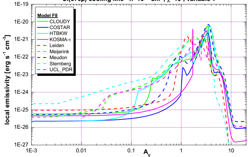
Cl(370 \mu ) cooling line - n=10^{5.5} cm ^{-3} , \chi=10^5 , variable T
