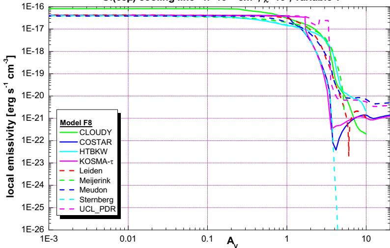
OI(63 \mu ) cooling line - n=10^{5.5} \text{ cm}^{-3} , \chi=10^5 , variable T
